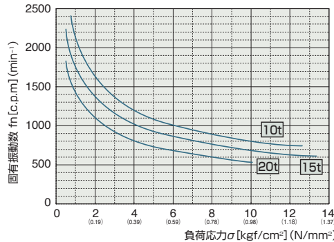
● 図2 固有振動数～応力特性
