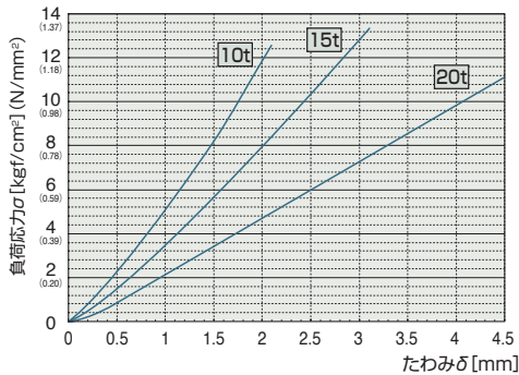
● 図1 応力～たわみ特性
